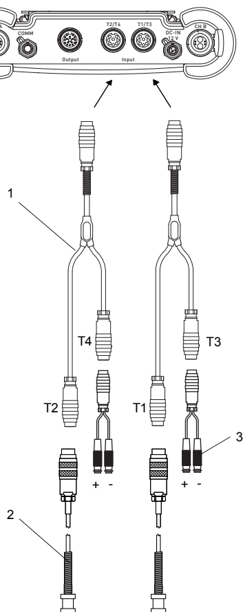
Рис. 7.9: Комбинированное измерение температуры, напряжения и тока (пример)
