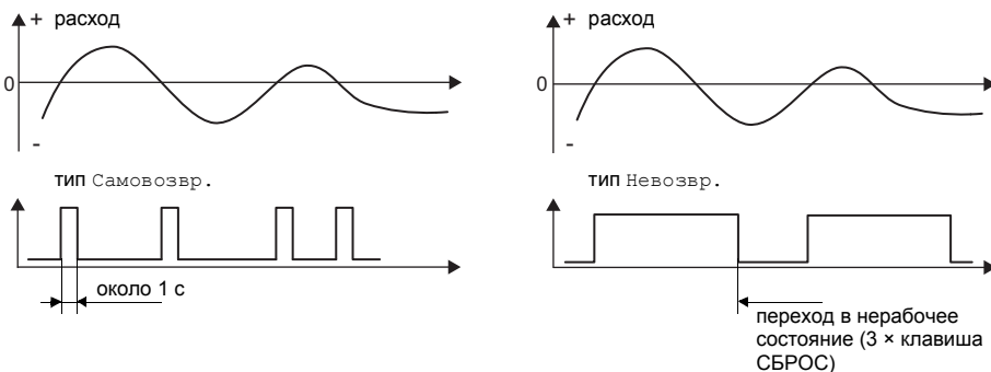
Рис. 17.1: Поведение реле при изменении направления потока
