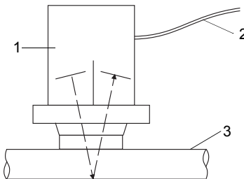
Рис. 20.1: Принцип измерения
