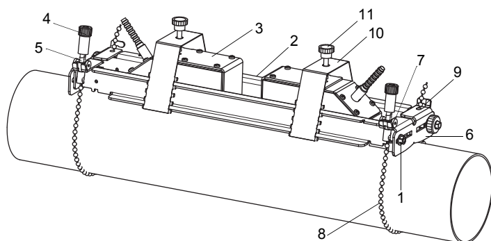
Рис. 6.15: Портативное монтажное крепление с цепями
