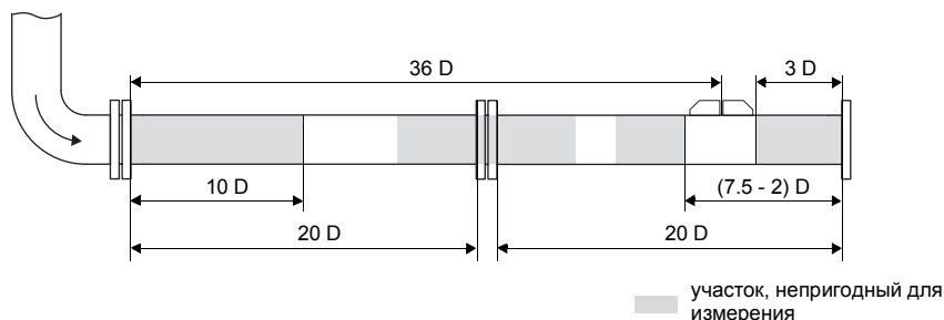
Рис. 3.12: Участок для места измерения с пригодным профилем потока и малым влиянием звуковых помех
