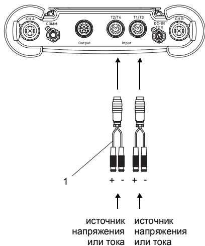
Рис. 7.8: Подключение 1 или 2 источника напряжения или тока
