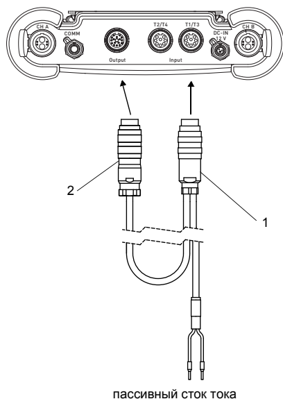
Рис. 7.10: Подключение адаптера для активного токового входа
